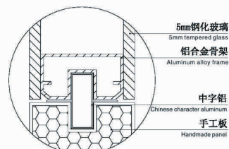
使用中字铝连接手工板 Using Chinese aluminum to connect handmade boards
