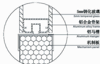
使用铝马槽连接机制板 Using aluminum manger to connect machine panels
